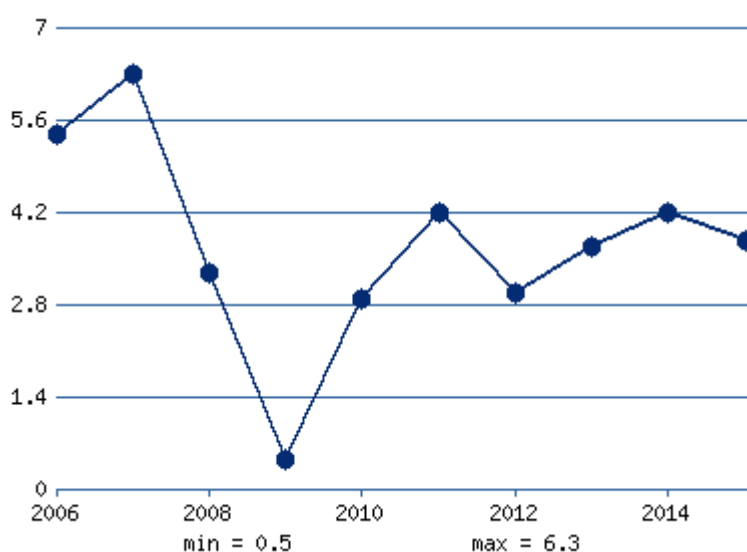
Рисунок – График «Темпы роста ВВП Гватемалы» (Сайт Мирровая экономика. Экономика Гватемалы [Электронный ресурс ]
