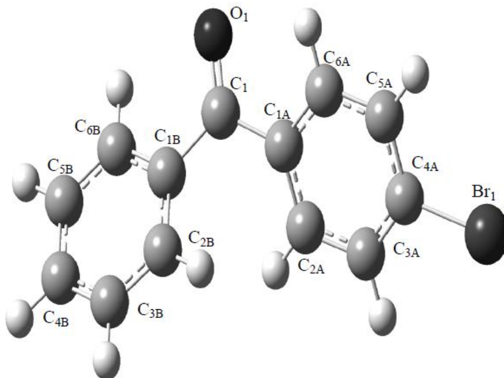
Рисунок 1 - Структура молекулы 4-ББФ по результатам моделирования
