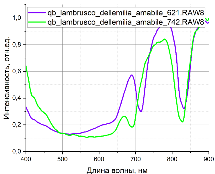
Рисунок 2. Спектр пропускания Образца №5. Цифрами обозначен номер используемого волновода, младшее число относится к дате 26.04.2022, старшее к 05.05.2022.
