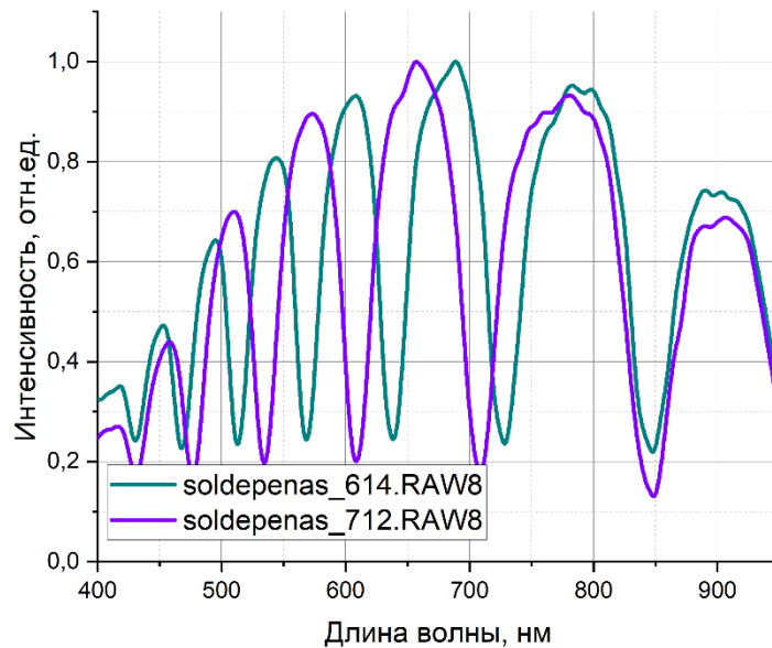
Рисунок 3. Спектр пропускания Образца №3. Цифрами обозначен номер используемого волновода, младшее число относится к дате 26.04.2022, старшее к 05.05.2022.
