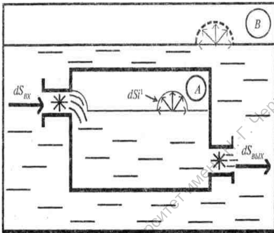
Рис.5. Энтропийные потоки в открытой системе (по Пригожину):
