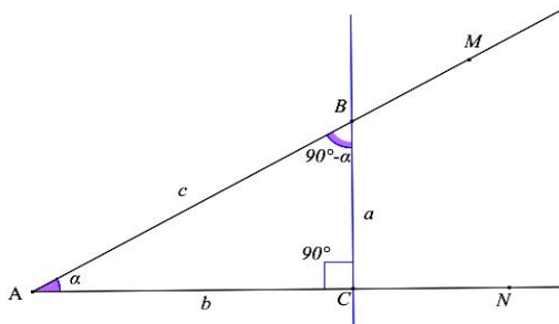
Рисунок 1. Обозначение сторон и углов в прямоугольном треугольнике
