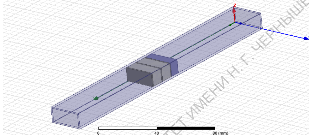
Рис. 1 Построение фотонной структуры относительно центрального нарушенного слоя
