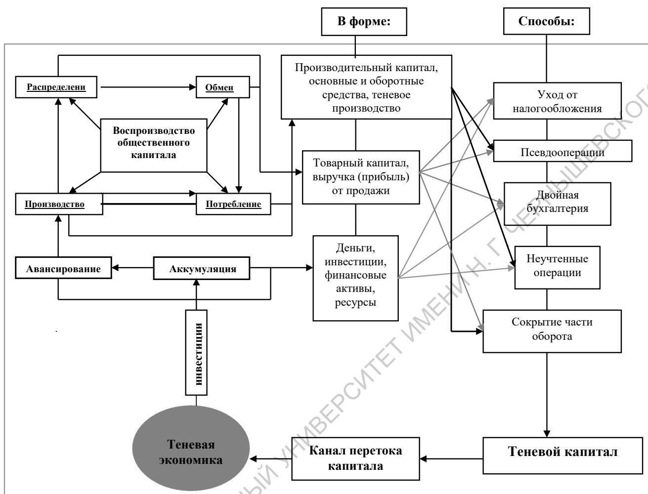
Рис. 13. Механизм перетока капитала в теневую экономику
