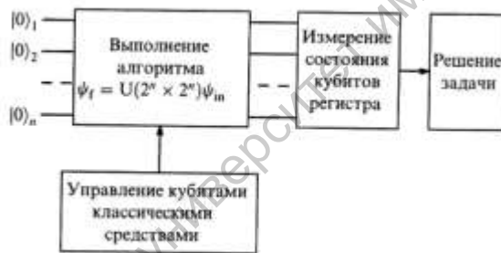
Рис. 7.4. Схема квантового компьютера
