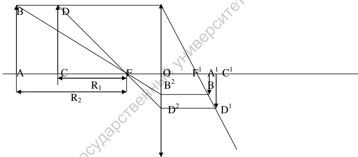
Рис. 1.3. Рисунок, иллюстрирующий обратную пропорциональность размера изображения расстоянию до объекта
