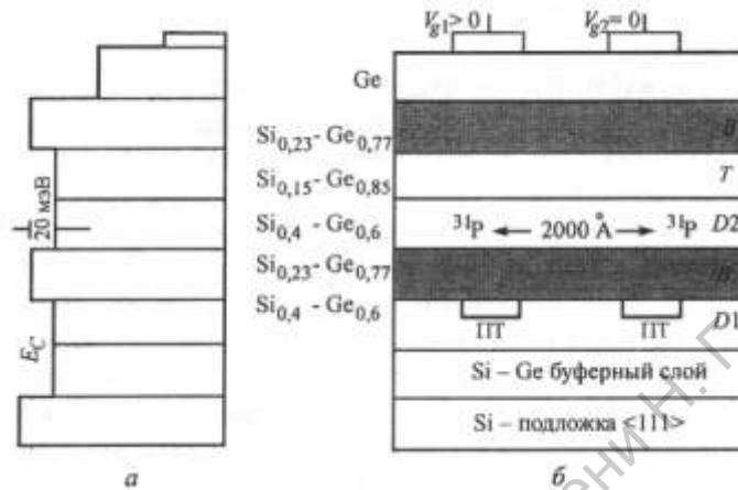
Рис. 7.6. Строение ячейки электронного спинового резонанса, состоящей из двух кубитов: а – энергетический профиль гетероструктуры Ge_{1-x}Si_x ; и – поперечный разрез двухкубитовой ячейки
