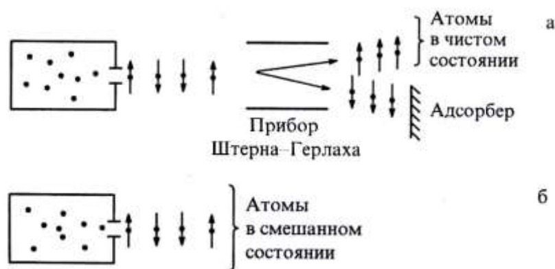
Рис. 7.5. Схема приготовления атомов в чистом (а) и смешанном (б) состояниях
